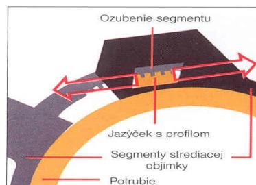
Obr. 2 Priečny rez
