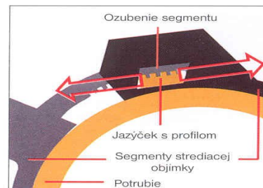
Obr. 2 Pričný rez
